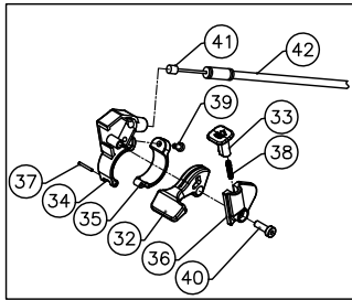
撥桿組詳圖
